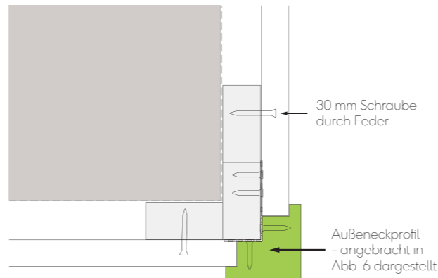
Abb. 7 - Details der Innenecke
