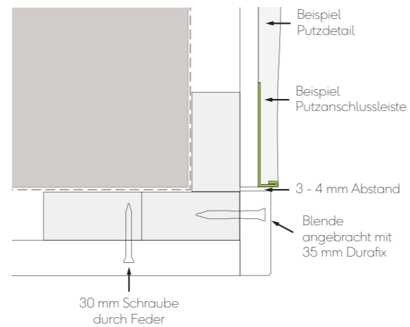
Abb. 20 - Eckprofil stößt an der Außenecke an den Putz an
