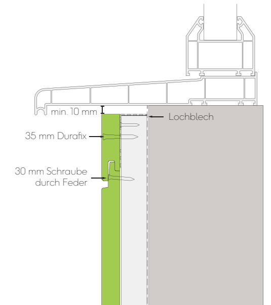
Abb. 3 - Detail Fenster/Türschwelle
