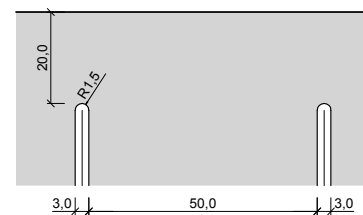
Ansicht "V-Fuge"
